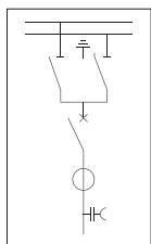
断路器柜
