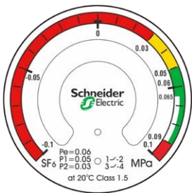
气体压力监测装置
