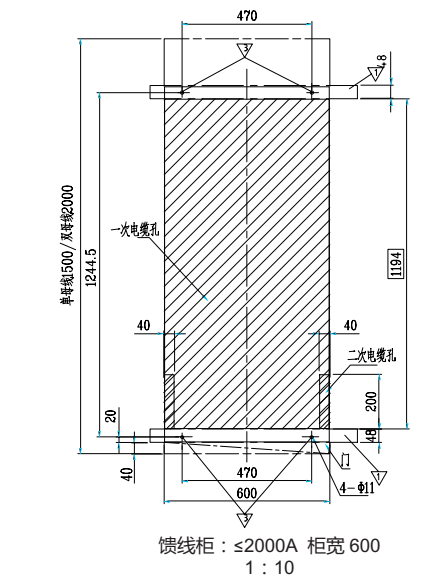
土建工程空间分布图
