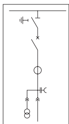
断路器柜
