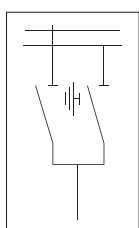
隔离柜
