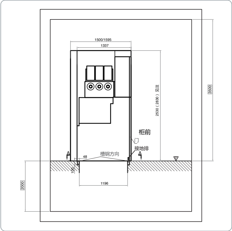
土建工程空间分布图
